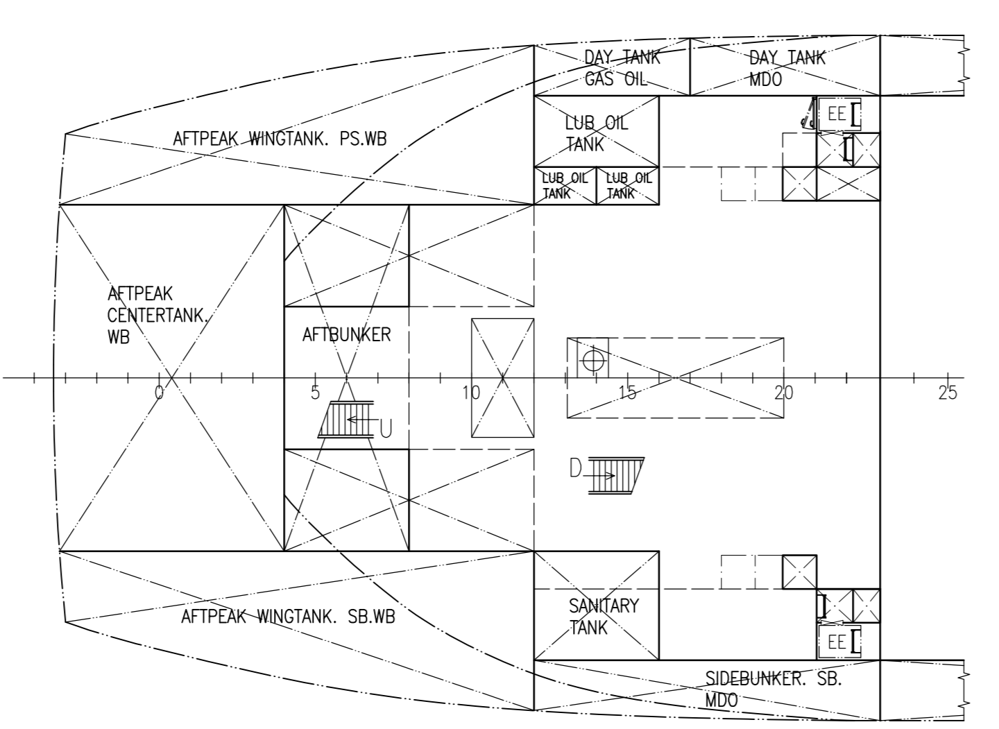
TWEEN DECK
